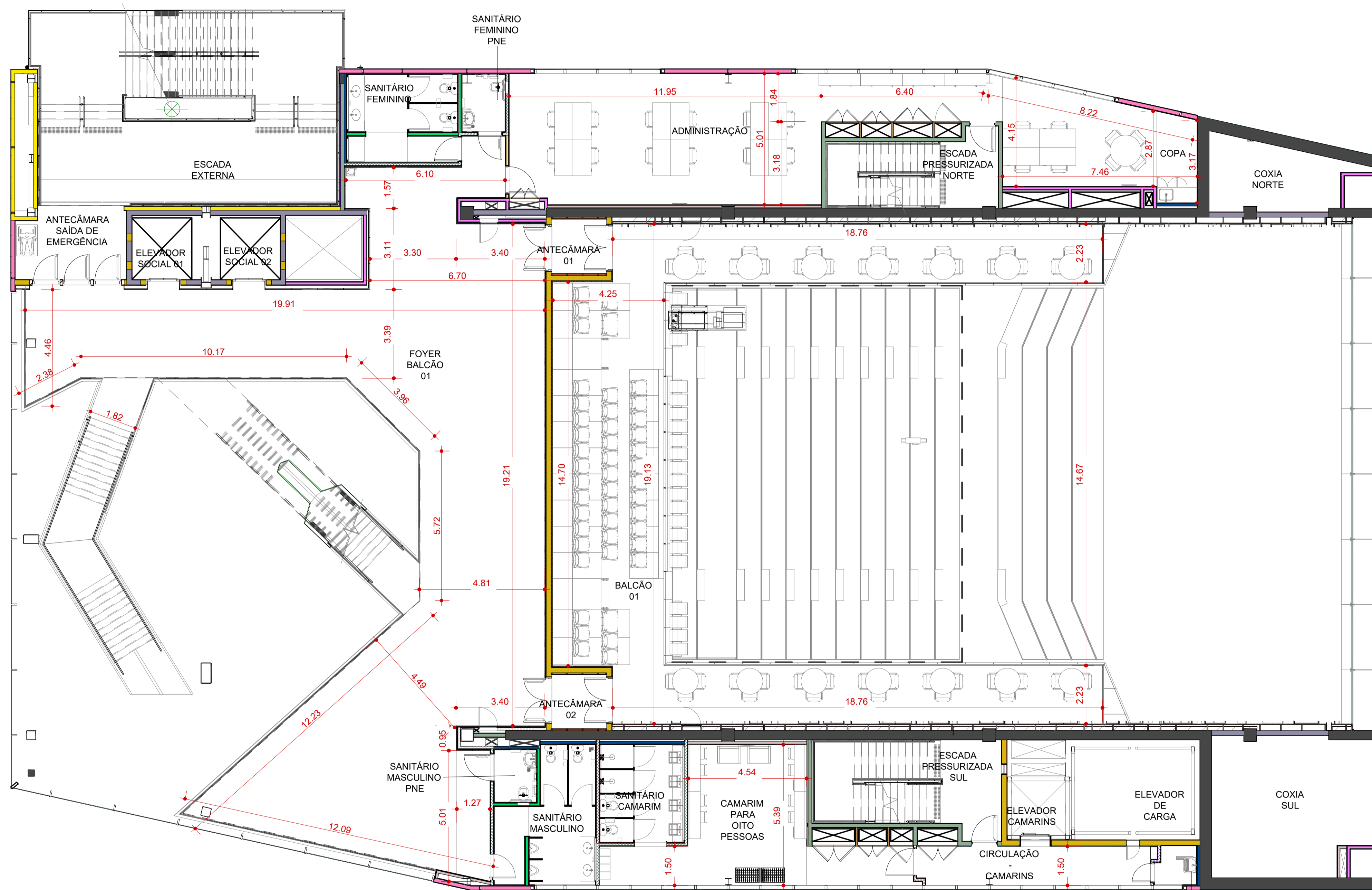
PLANTA BAIXA - NÍVEL DO BALÇÃO 01 ESCALA 1:100 MEDIDAS EM METROS (m)
