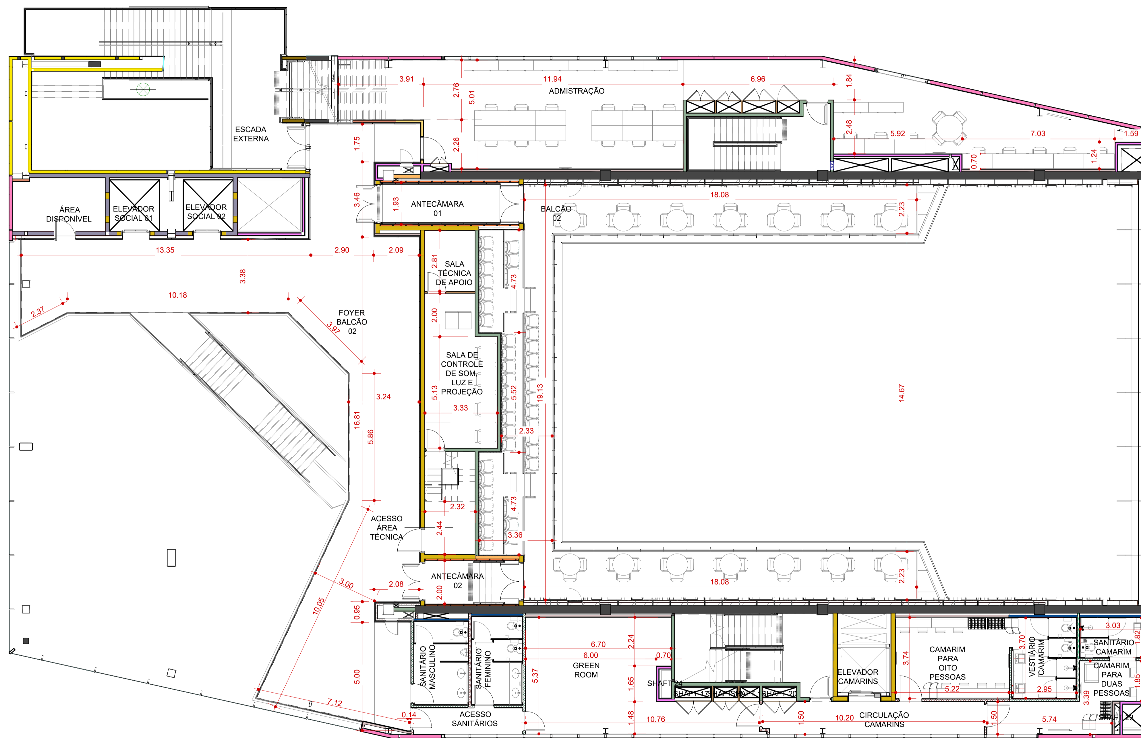
PLANTA BAIXA - NIVEL DO BALCÃO 02 ESCALA 1:100 MEDIDAS EM METROS (m)
